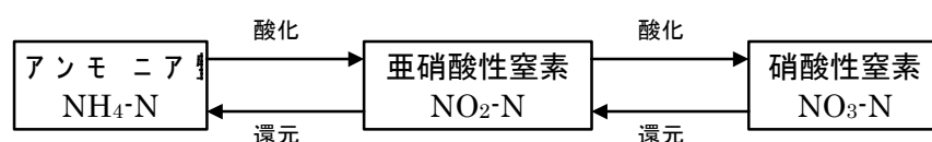
図-1 水中での窒素の形態変化
