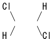
トランス異性体
