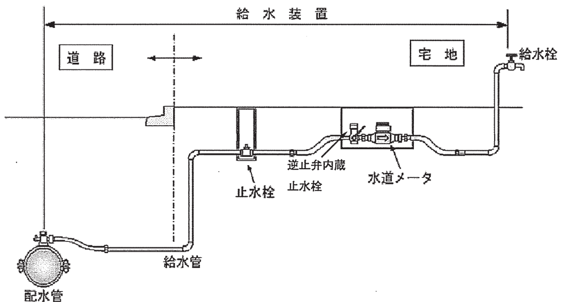
給水装置の概念図の一例
